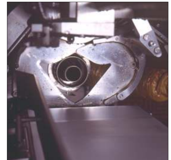
Verdrängerschere mit großem Durchlass Displacer with large passage Pincas de desplazamiento a grand passage Chapa de desplazamiento con gran pasada
